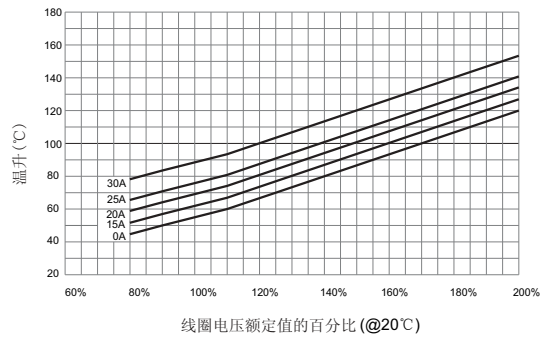
线圈温升
